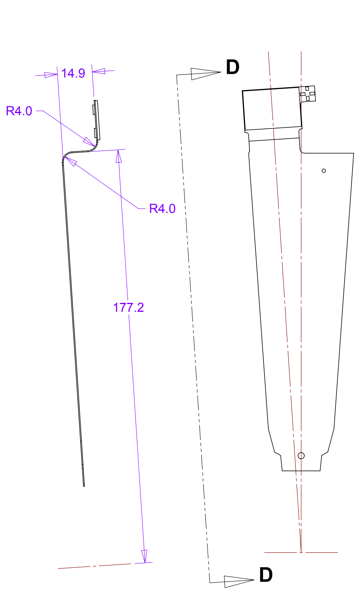
SECTION D-D
